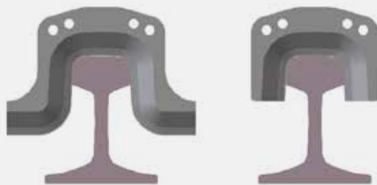
Режещ накрайник ФОРМА А (с шайгер)
